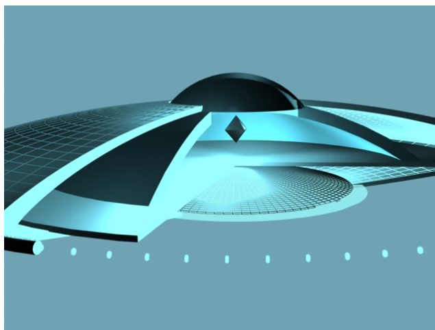
Quatre technologies : double rotor, supraconducteurs, oscillateur et tore.
