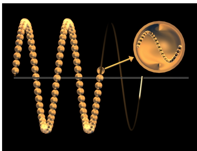
Les ondes sont des spires de temps. En zoomant sur un quantum de temps on aperçoit une autre série de chronons, et ainsi de suite.
