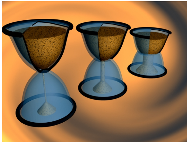
Dans la réalité, le sable s'écoule à des vitesses différentes. La densité de temps augmente quand l'espace diminue.
