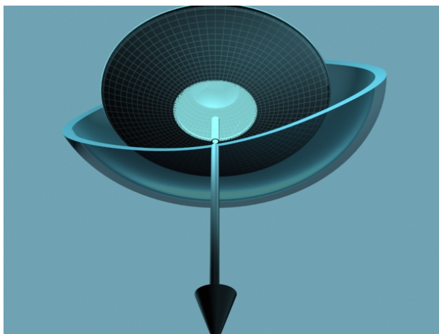
La gravitation potentielle (flèche) est annulée (tube sans direction au-dessus). La dégravitation croît comme le temps au carré.
