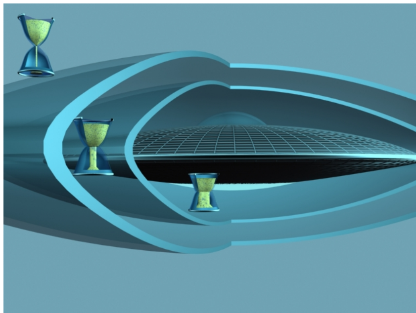
Un vaisseau est entouré de couches différentes d'écoulements temporels.
