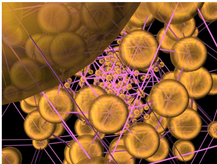
Une perspective permet une meilleure visualisation de la superposition du temps quantique. L'écoulement du temps vient des intervalles d'inexistence temporelle (traits mauves) dans les sphères concentriques de l'univers.
