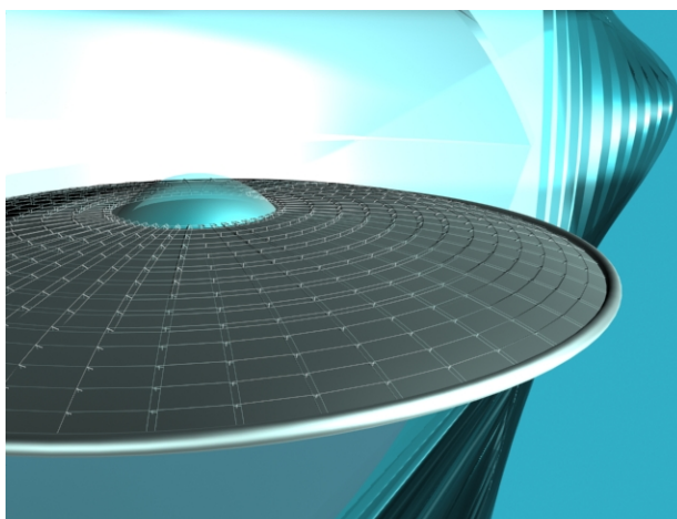
Il n'existe pas de couche limite sur laquelle l'onde choc pourrait naître.
